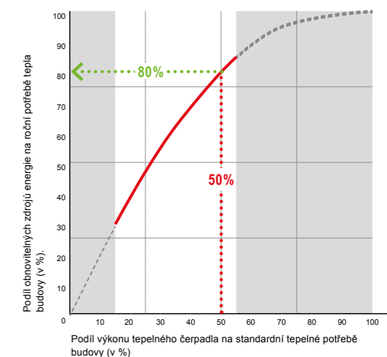
Při 50% tepelné zátěži zajistí Belaria® fit 80% roční spotřeby energie. Ve výsledku tak lze splnit zákonné požadavky na vysoký podíl obnovitelných zdrojů energie, nákladově efektivní, a to i ve velkých objektech.
